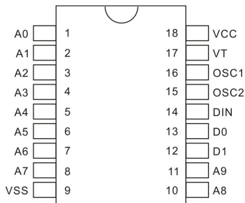
PT2272A-M2
