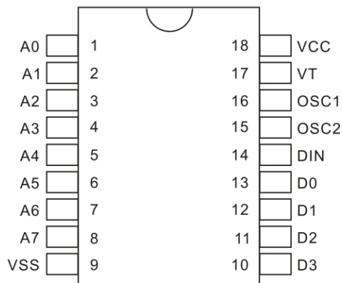
PT2272-M4/L4
