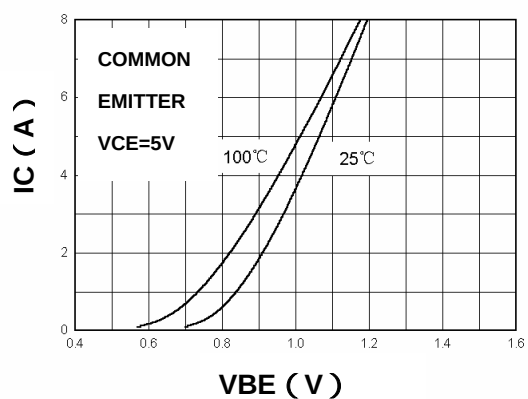
IC - VBE
