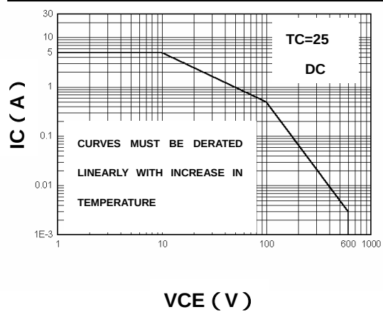
SOA
