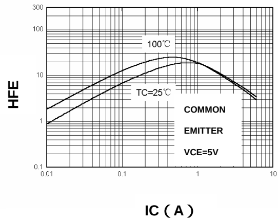
HFE - IC
