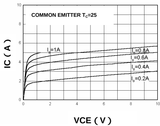
IC - VCE
