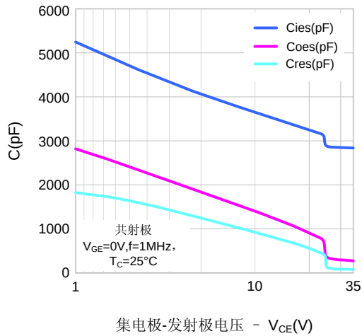
图7. 电容特性
