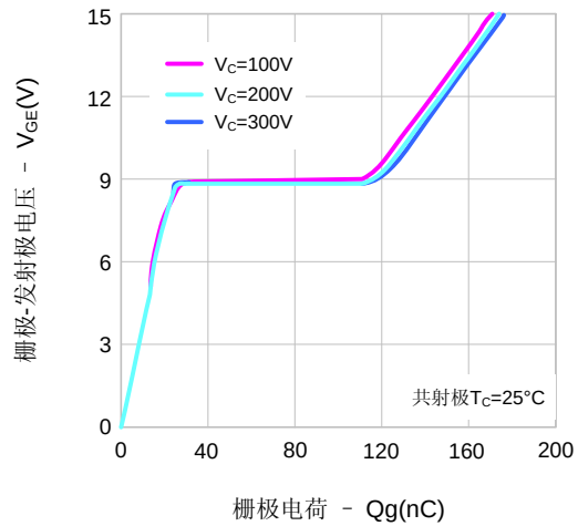
图8. 栅极电荷
