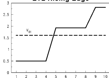
ETL Rising Edge
