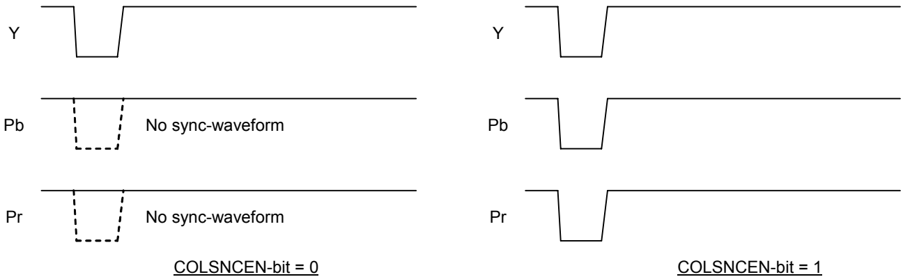
Fig. 119 525i / 625i / 525p / 625p case
