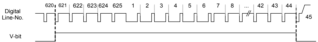
Fig. 59 625p case
