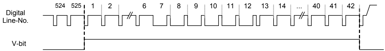
Fig. 58 525p case
