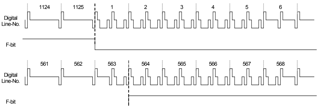
Fig. 57 1080i mode
