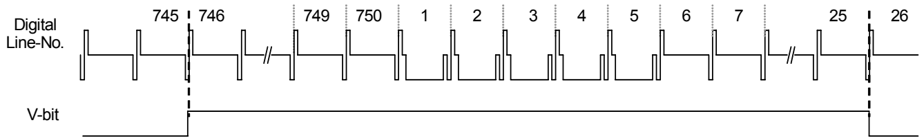
Fig. 60 720 case
