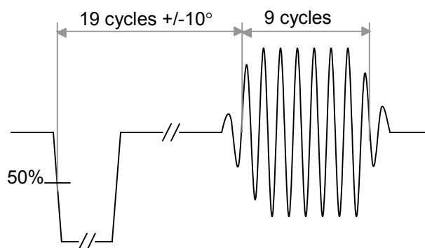
Fig. 163 NTSC Color Burst
