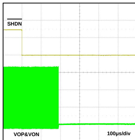
关断时序
