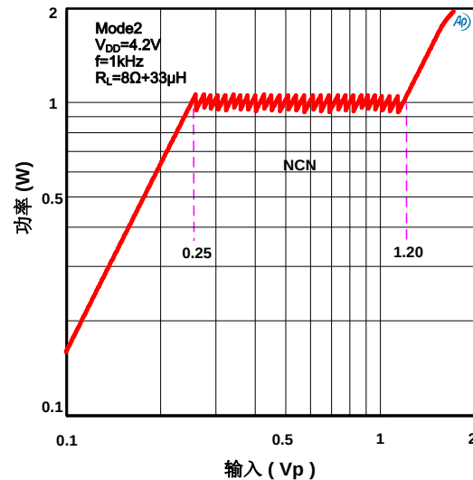
功率 vs 输入
