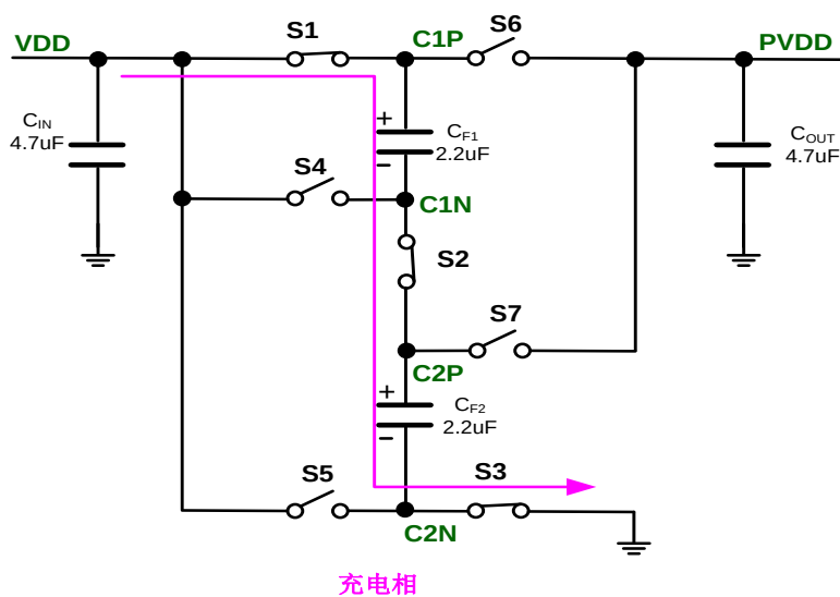
图 10 Φ1: Flying 电容充电
