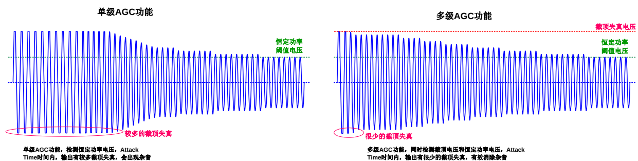
图 9 单级 AGC/多级 AGC 工作原理图
