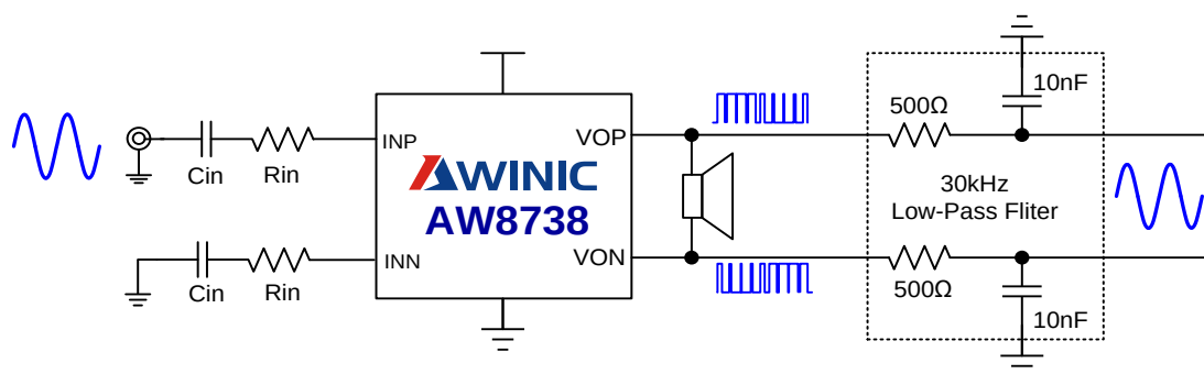
图 6 AW8738 测试电路图
