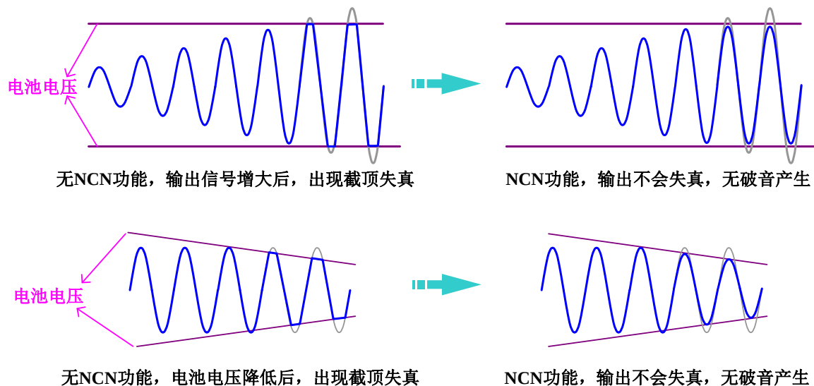
图 7 传统 NCN 工作原理图
