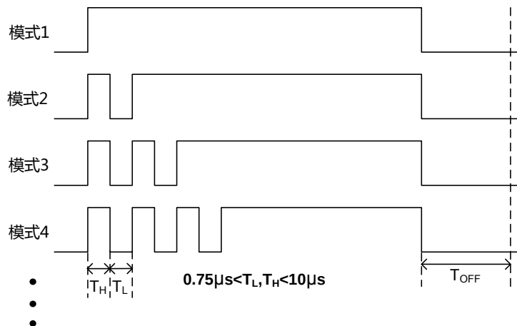
图 14 一线脉冲控制方法
