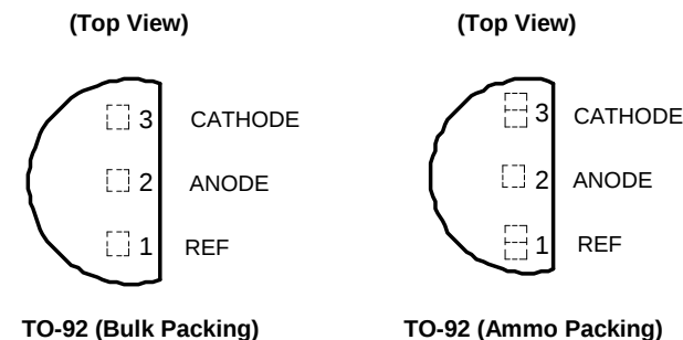
TO-92 (Bulk Packing)
