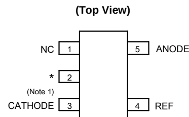
SOT-23-5
