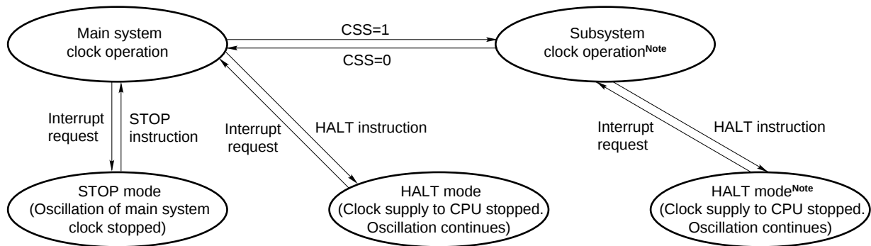
Fig. 7-1 Standby Function
