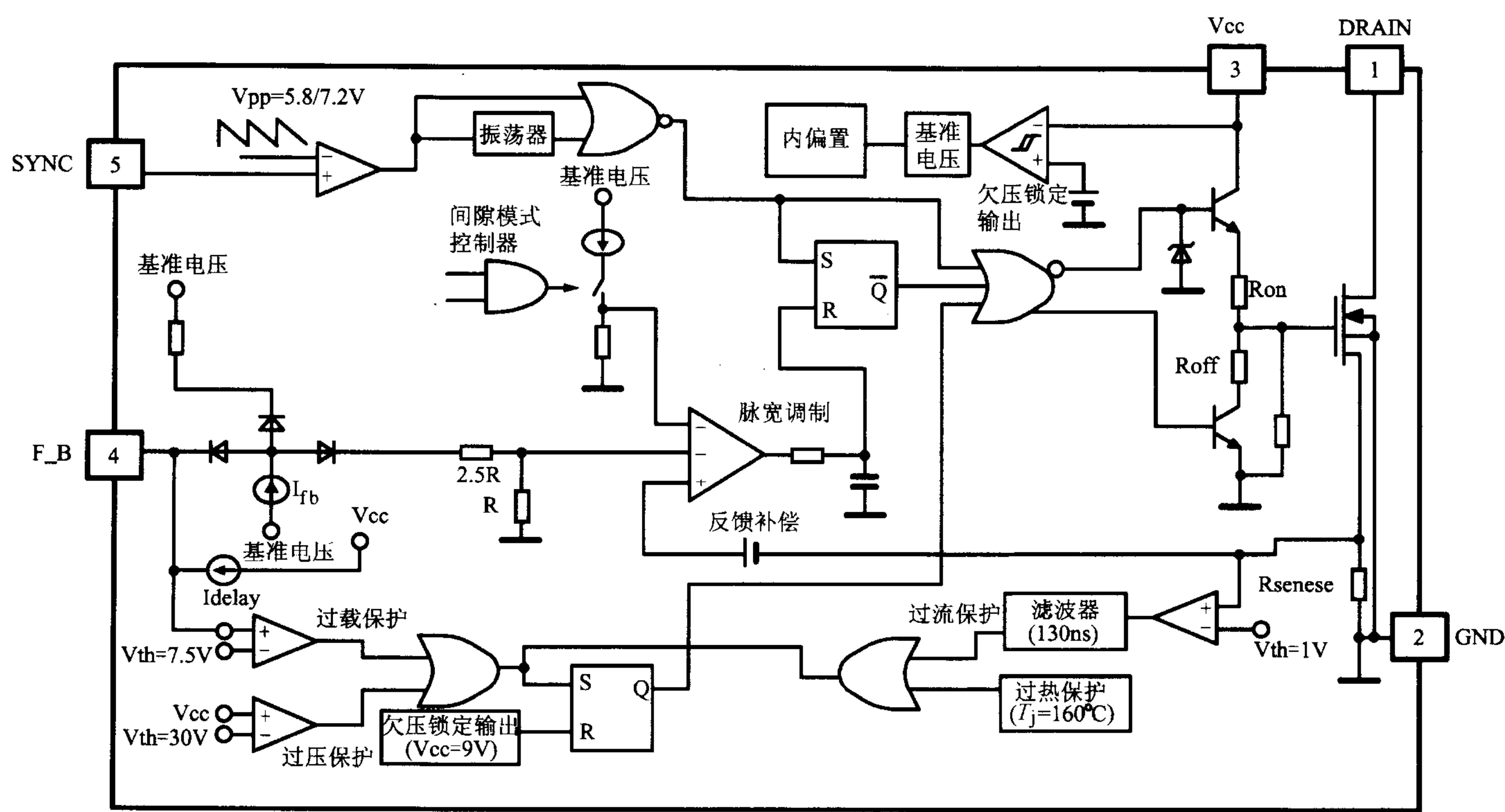
图 36 DP904C 内部等效图
