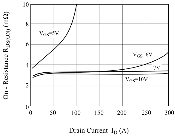
Fig7. R_{DS(ON)} - I_D
