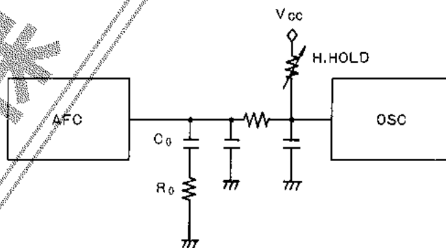
Fig 5 基本回路
