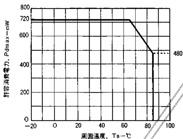
Pdmax-Ta特性
