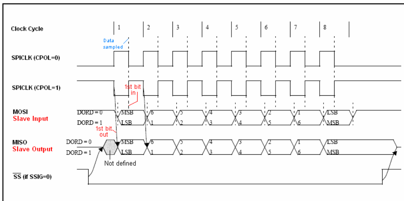
图 14-6. SPI从机传送,CPHA=1
