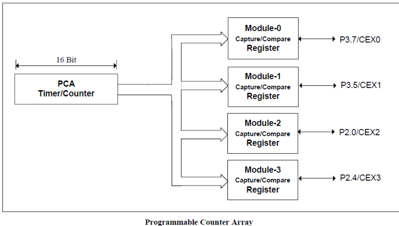
图13-1. PCA 方框图
