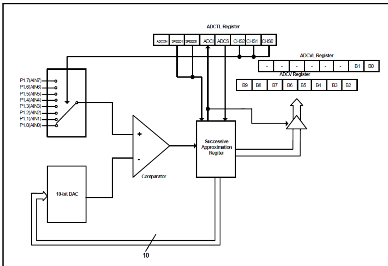
图 15-1. ADC功能框图
