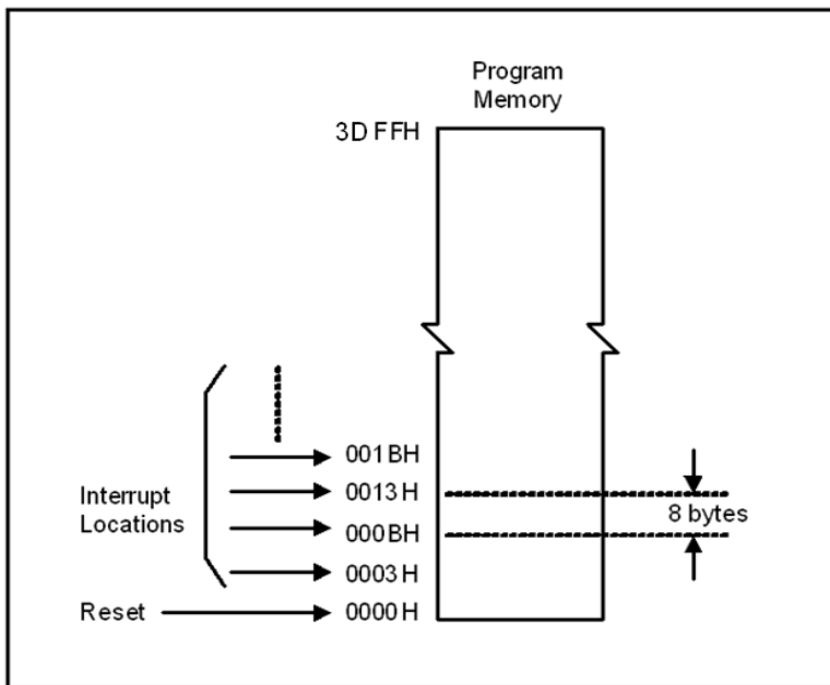
图 8-1 程序存储器
