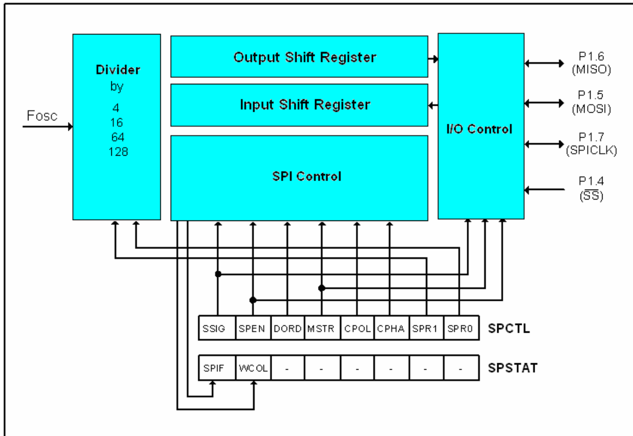
图 14-1. SPI 框图
