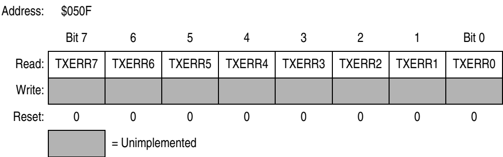
Figure 23-25. Transmit Error Counter (CTXERR)
