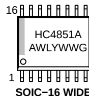
SOIC-16 WIDE
