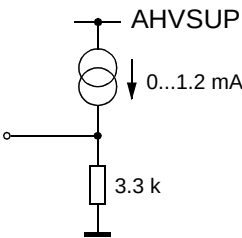
Fig. 4-21: Output Pins: DACM_R/L
