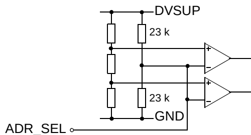
Fig. 4-16: Input Pin: ADR_SEL
