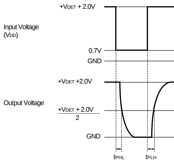
CMOS Output
