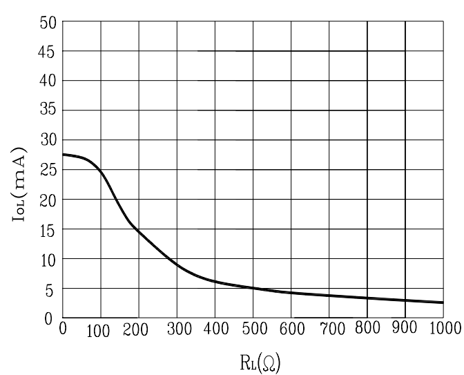
Fig. 4 I_{OL}-R_L
