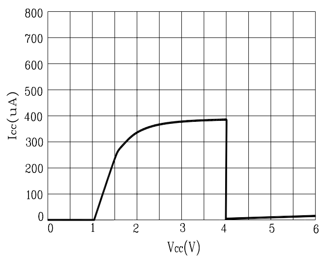
Fig. 2 I_{CC}-V_{CC}
