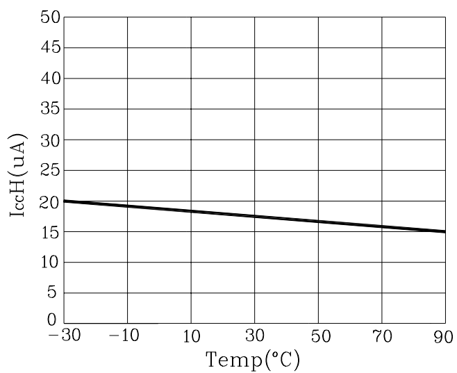
Fig. 3 I_{CCH}-Temp
