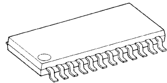
SSOP24-P-300-1.00
