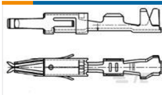
TE Part #962876-3 MT2 REC 1.6 Contact SWS Au
