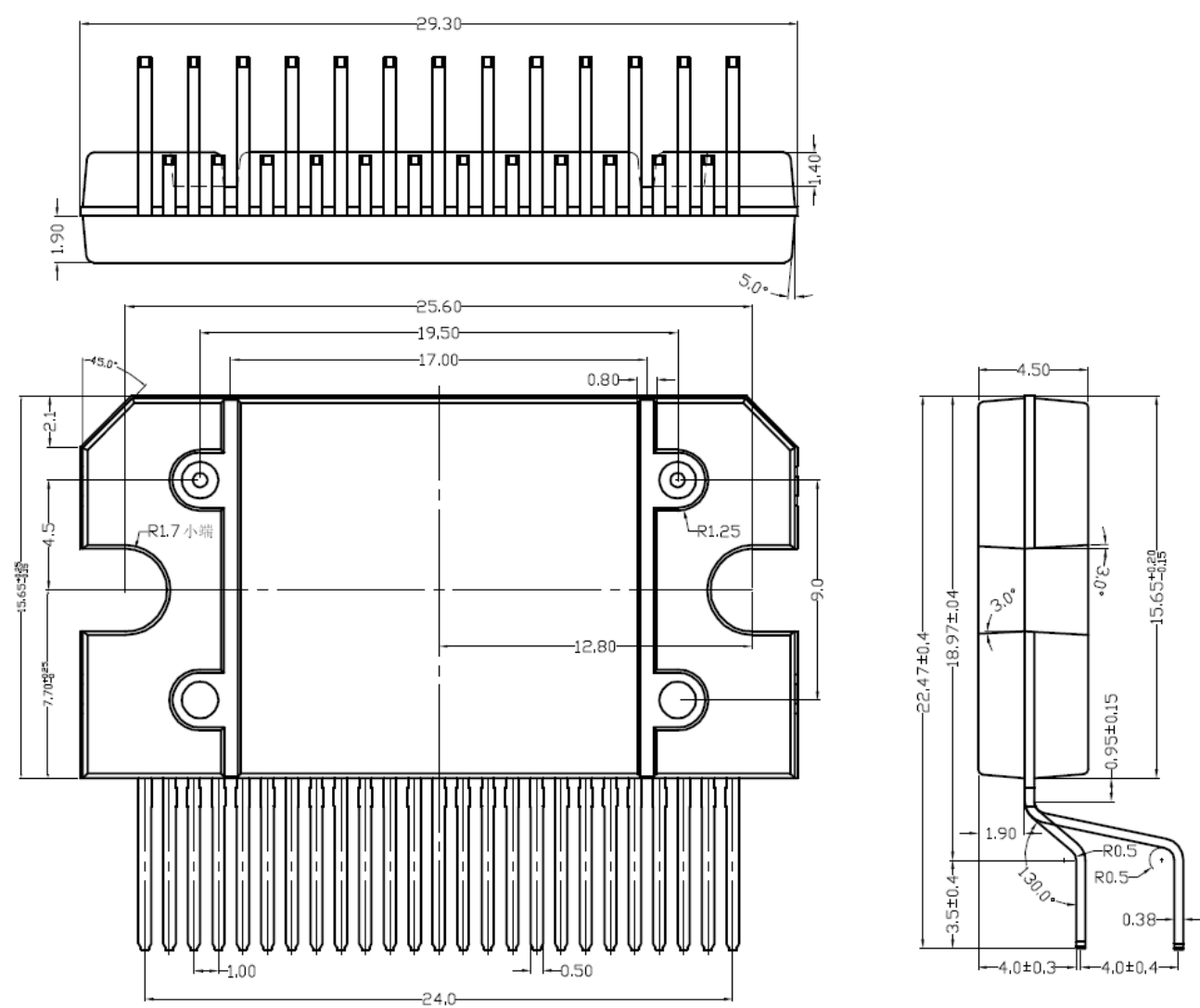
封装外形图： （单位:毫米）
